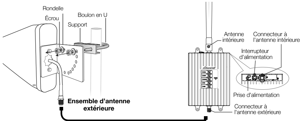
Diagramme de composants de l'amplificateur
