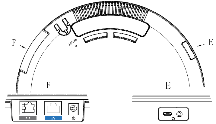
Kaskadierer-Port LAN Anschluss Strom
